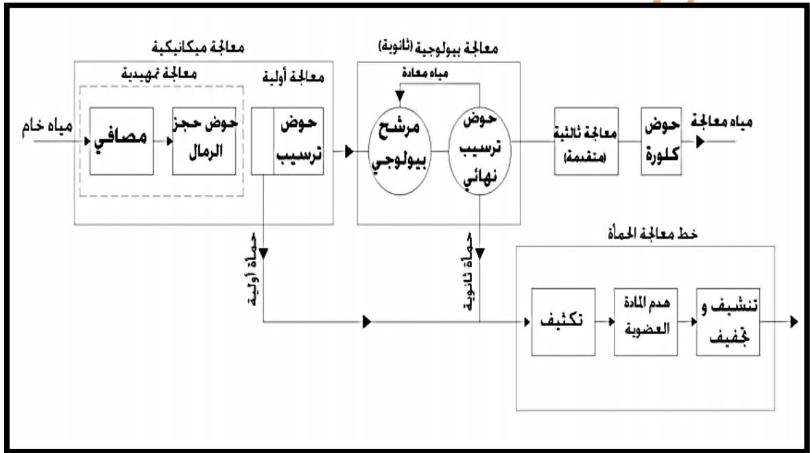
مخطط معالجة مياه المجاري (البلدية)
